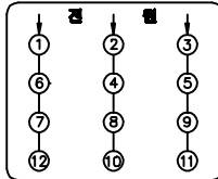
Δ 결선(440V)
