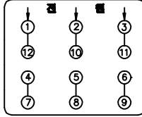
Δ 결선(440V)
