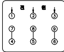
Δ 결선(440V)
