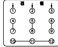
Y 결선(440V)
