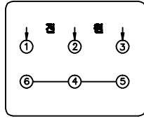
Y 결선(380V)
