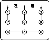
Δ 결선(220V)
