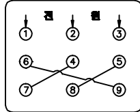
Δ 결선(440V)
