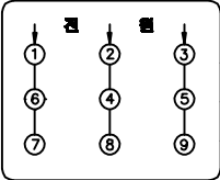
Δ 결선(220V)
