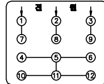
Y 결선(440V)
